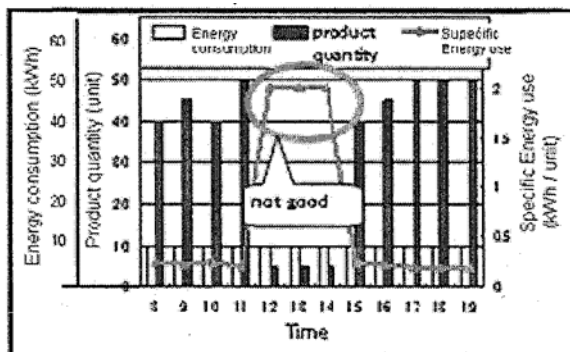
Рис. А.2 – Изменения индикаторов энергоэффективности (удельное потребление энергии: кВтч/ед. продукции)
